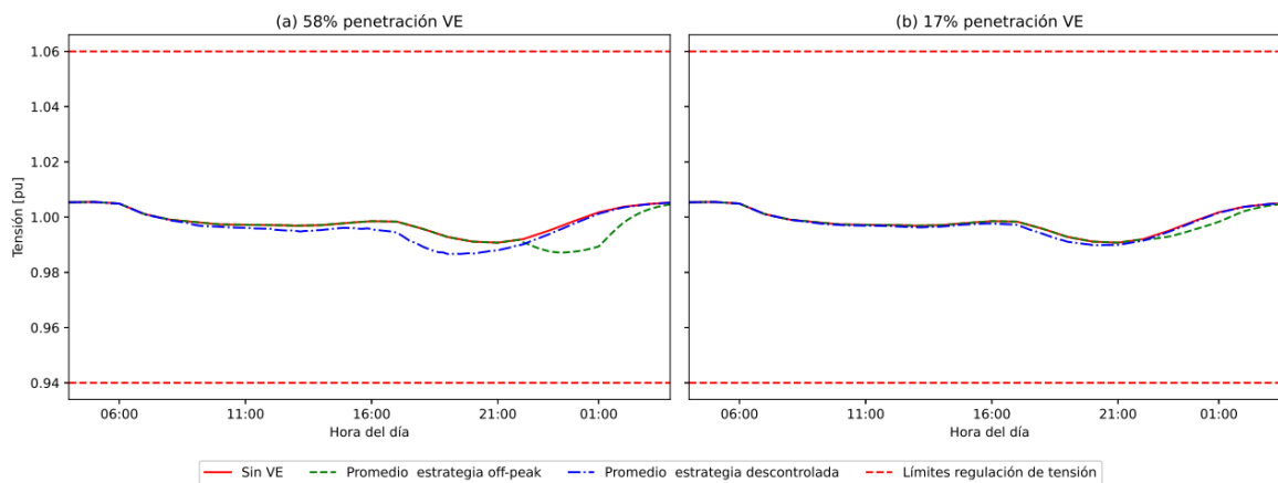
Figura 41: Comparación de la tensión eléctrica en el nodo 4 cuando los VE tienen acceso solamente a cargadores domiciliarios y de CCR. (Fuente: Elaboración propia).
