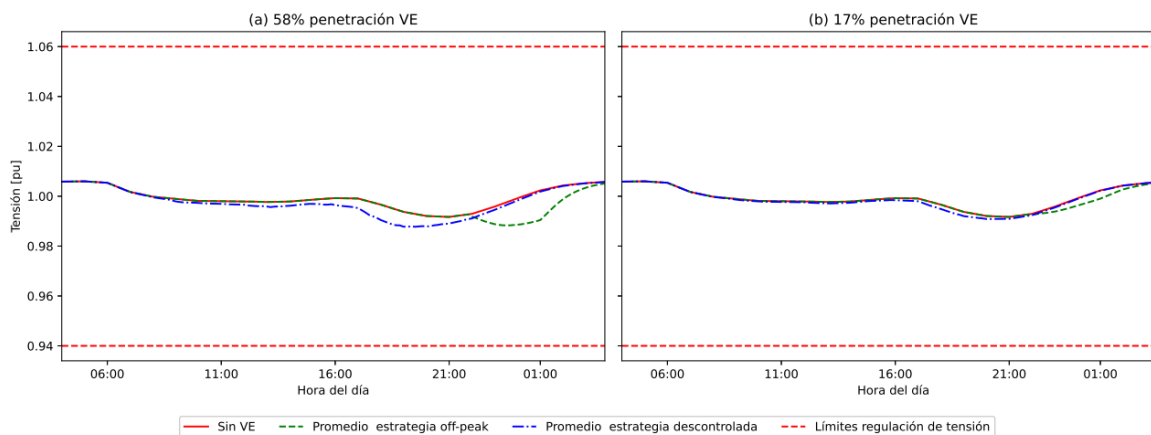
Figura 39: Comparación de la tensión eléctrica en el nodo 3 cuando los VE tienen acceso solamente a cargadores domiciliarios y de CCR. (Fuente: Elaboración propia).
