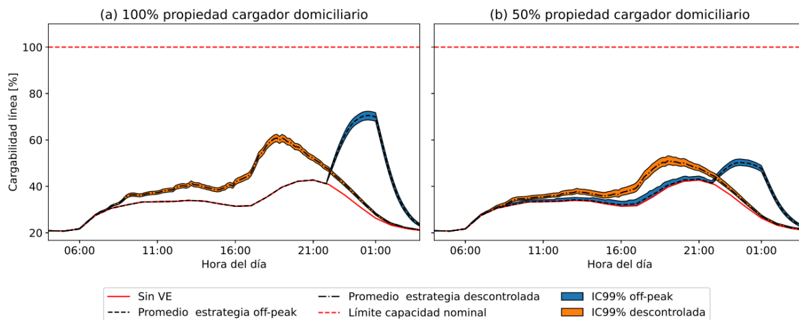
Figura 56: Comparación de la sobrecarga de la línea 2 cuando los VE tienen acceso solamente a cargadores domiciliarios y de CCR. (Fuente: Elaboración propia).
