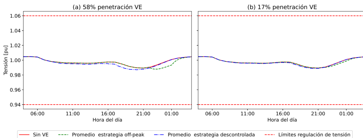
Figura 17: Comparación de la tensión eléctrica en el nodo 1 cuando los VE tienen acceso a carga en todos los estados de estacionamiento. (Fuente: Elaboración propia).
