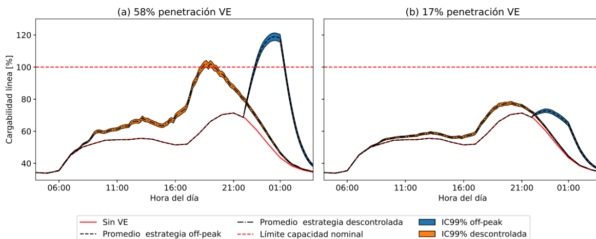
Figura 18: Comparación de la sobrecarga de la línea 1 cuando los VE tienen acceso solamente a cargadores domiciliarios y de CCR. (Fuente: Elaboración propia).
