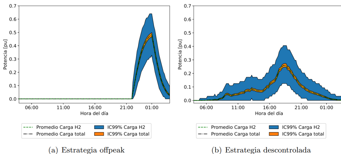
Figura 34: Comparación de patrones de carga domiciliarios de VE normalizados en función de la potencia instalada para una penetración del 17% en la carga H2 y el total del alimentador para una penetración del 58% (Fuente: Elaboración propia).
