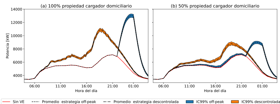
Figura 20: Comparación de la demanda eléctrica en cabecera del alimentador con un 58% de penetración, considerando que los VE tienen acceso solamente a cargadores domiciliarios y de CCR. (Fuente: Elaboración propia).
