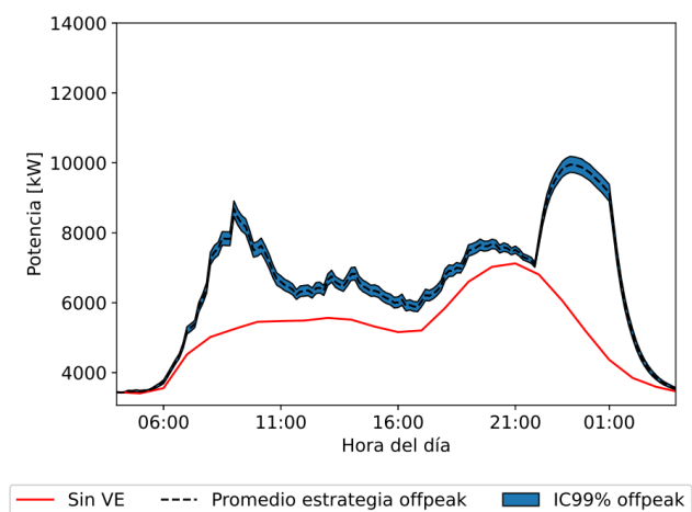
Figura 61: Demanda eléctrica producto de todos los eventos de carga de la flota de VE simulada para el escenario 4. (Fuente: Elaboración propia).
