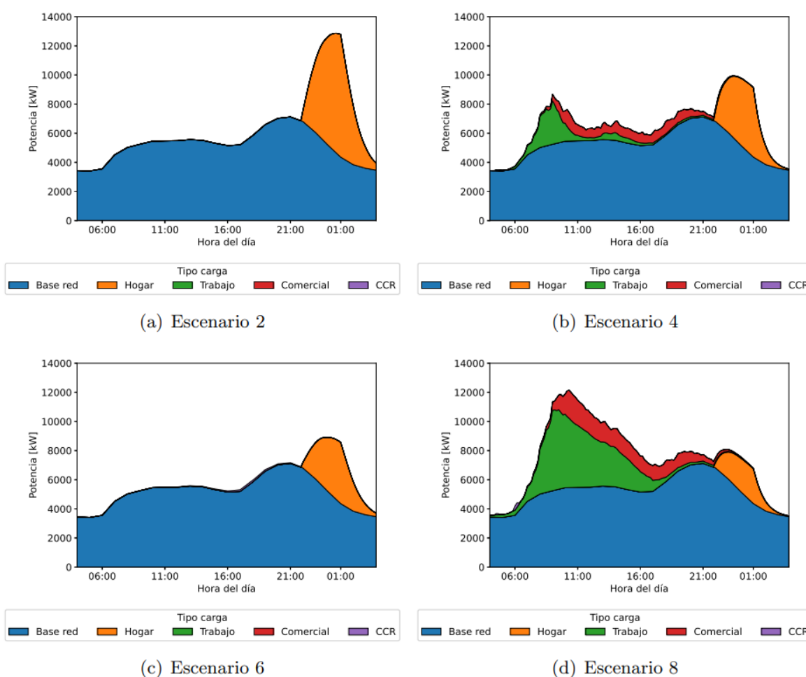
Figura 31: Comparación de escenarios 2, 4, 6 y 8 de la demanda eléctrica promedio de todos los eventos de carga bajo una estrategia offpeak. (Fuente: Elaboración propia).
