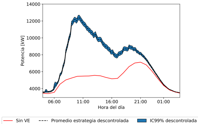
Figura 64: Demanda eléctrica producto de todos los eventos de carga de la flota de VE simulada para el escenario 7. (Fuente: Elaboración propia).
