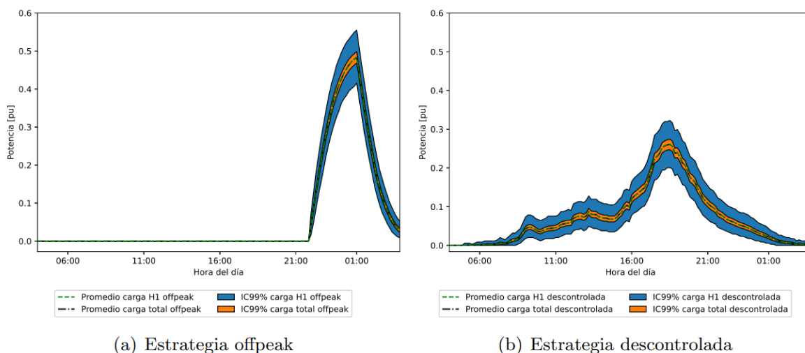
Figura 33: Comparación de patrones de carga domiciliarios de VE normalizados en función de la potencia instalada para una penetración del 58% (Fuente: Elaboración propia).
