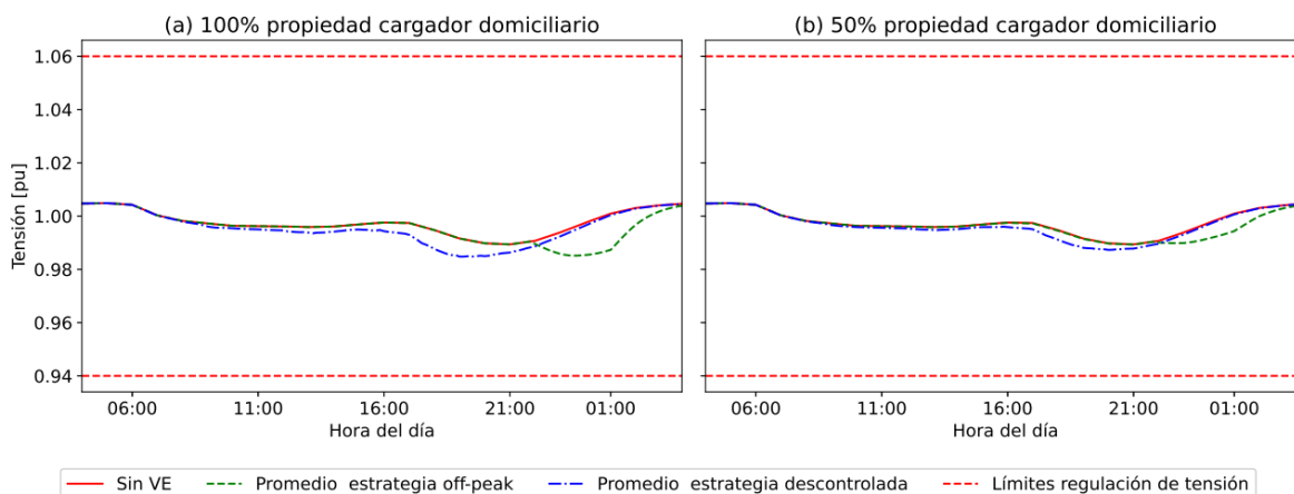
Figura 22: Comparación de la tensión eléctrica en el nodo 1 para un 58% de penetración cuando los VE tienen acceso solamente a cargadores domiciliarios y de CCR. (Fuente: Elaboración propia).
