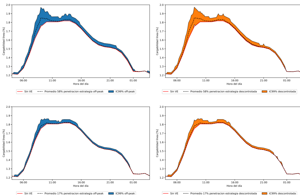
Figura 53: Comparación ante distintos escenarios de la sobrecarga de la línea 5 que abastece al consumo de lugar de trabajo. (Fuente: Elaboración propia).
