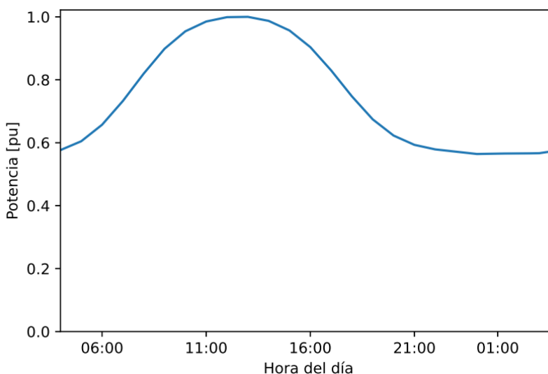
Figura 13: Perfil diario de demanda aplicado a todas las cargas de carácter comercial en el alimentador. (Fuente EPRI [60])
