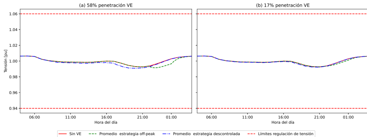
Figura 46: Comparación de la tensión eléctrica en el nodo 6 cuando los VE tienen acceso a carga en todos los estados de estacionamiento. (Fuente: Elaboración propia).
