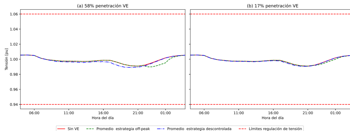
Figura 38: Comparación de la tensión eléctrica en el nodo 2 cuando los VE tienen acceso a carga en todos los estados de estacionamiento. (Fuente: Elaboración propia).
