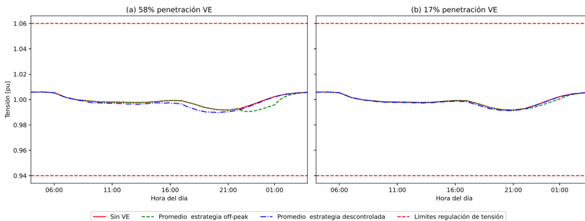
Figura 40: Comparación de la tensión eléctrica en el nodo 3 cuando los VE tienen acceso a carga en todos los estados de estacionamiento. (Fuente: Elaboración propia).
