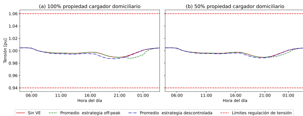
Figura 23: Comparación de la tensión eléctrica en el nodo 1 para un 58% de penetración cuando los VE tienen acceso a carga en todos los estados de estacionamiento. (Fuente: Elaboración propia).
