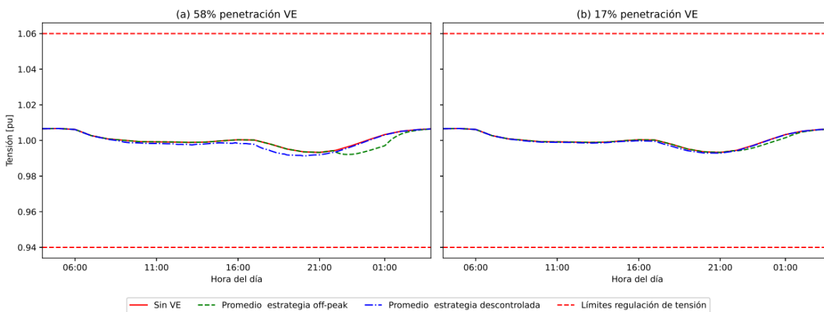
Figura 44: Comparación de la tensión eléctrica en el nodo 5 cuando los VE tienen acceso a carga en todos los estados de estacionamiento. (Fuente: Elaboración propia).
