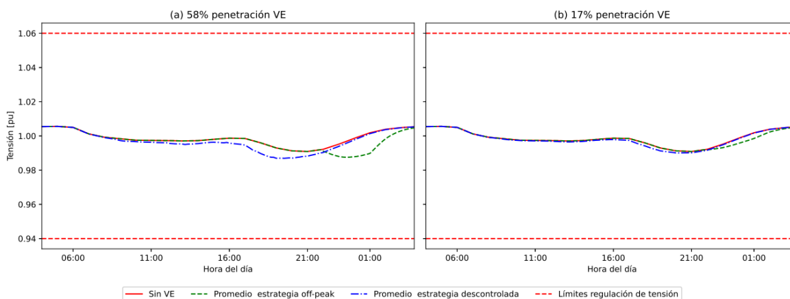
Figura 37: Comparación de la tensión eléctrica en el nodo 2 cuando los VE tienen acceso solamente a cargadores domiciliarios y de CCR. (Fuente: Elaboración propia).
