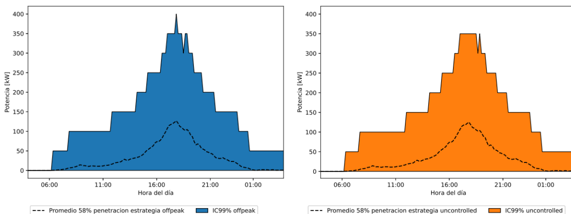
Figura 32: Patrones de carga de VE en CCR para una penetración del 58%, correspondiente a los escenarios 5 y 6. (Fuente: Elaboración propia).
