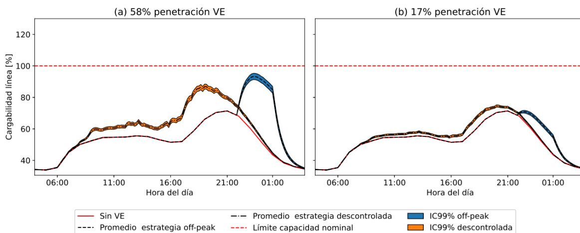
Figura 19: Comparación de la sobrecarga de la línea 1 cuando los VE tienen acceso a carga en todos los estados de estacionamiento. (Fuente: Elaboración propia).
