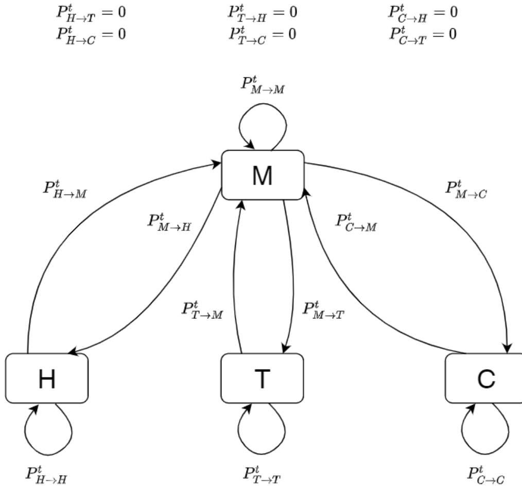
Figura 6: Diagrama Markov Chain de posibles transiciones de estado de VE para un instante t . (Fuente: Elaboración propia).
