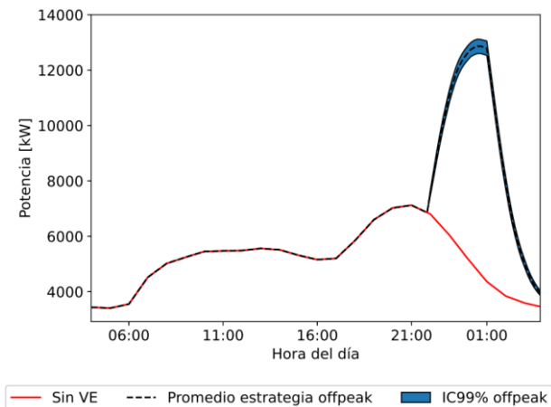
Figura 59: Demanda eléctrica producto de todos los eventos de carga de la flota de VE simulada para el escenario 2. (Fuente: Elaboración propia).
