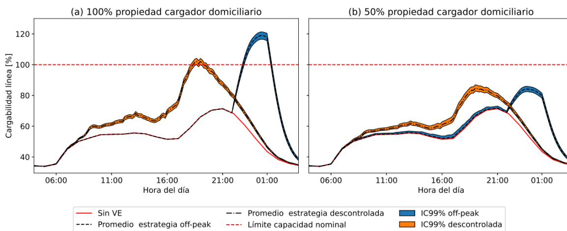
Figura 24: Comparación de la sobrecarga de la línea 1 cuando los VE tienen acceso solamente a cargadores domiciliarios y de CCR. (Fuente: Elaboración propia).
