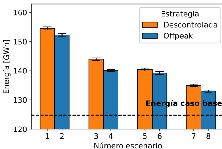
Figura 28: Comparación de la energía demandada diariamente producto de solo los eventos de carga en el alimentador para una penetración de VE del 58% (Fuente: Elaboración propia).
