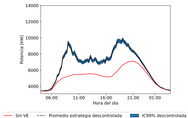
Figura 60: Demanda eléctrica producto de todos los eventos de carga de la flota de VE simulada para el escenario 3. (Fuente: Elaboración propia).
