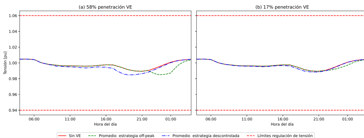
Figura 35: Comparación de la tensión eléctrica en el nodo 1 cuando los VE tienen acceso solamente a cargadores domiciliarios y de CCR. (Fuente: Elaboración propia).
