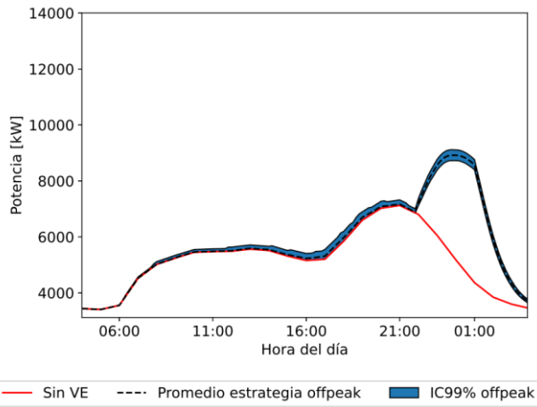
Figura 63: Demanda eléctrica producto de todos los eventos de carga de la flota de VE simulada para el escenario 6. (Fuente: Elaboración propia).
