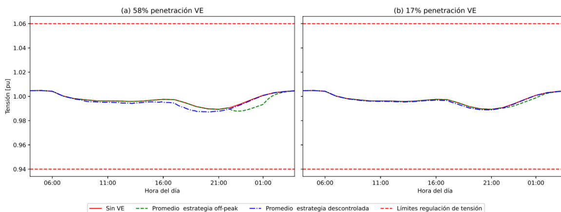
Figura 36: Comparación de la tensión eléctrica en el nodo 1 cuando los VE tienen acceso a carga en todos los estados de estacionamiento. (Fuente: Elaboración propia).
