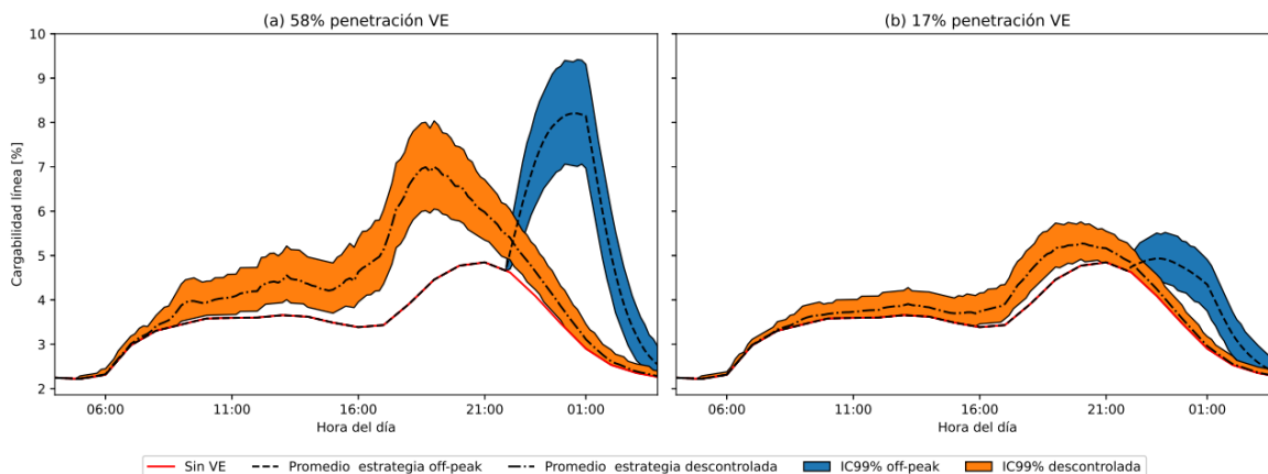
Figura 49: Comparación de la sobrecarga de la línea 3 cuando los VE tienen acceso solamente a cargadores domiciliarios y de CCR. (Fuente: Elaboración propia).
