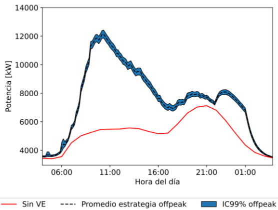
Figura 65: Demanda eléctrica producto de todos los eventos de carga de la flota de VE simulada para el escenario 8. (Fuente: Elaboración propia).
