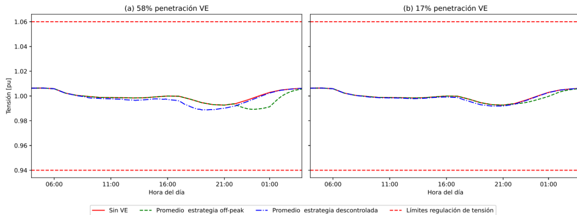
Figura 45: Comparación de la tensión eléctrica en el nodo 6 cuando los VE tienen acceso solamente a cargadores domiciliarios y de CCR. (Fuente: Elaboración propia).
