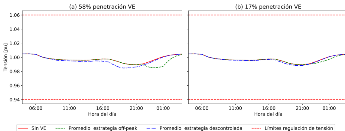
Figura 16: Comparación de la tensión eléctrica en el nodo 1 cuando los VE tienen acceso solamente a cargadores domiciliarios y de CCR. (Fuente: Elaboración propia).
