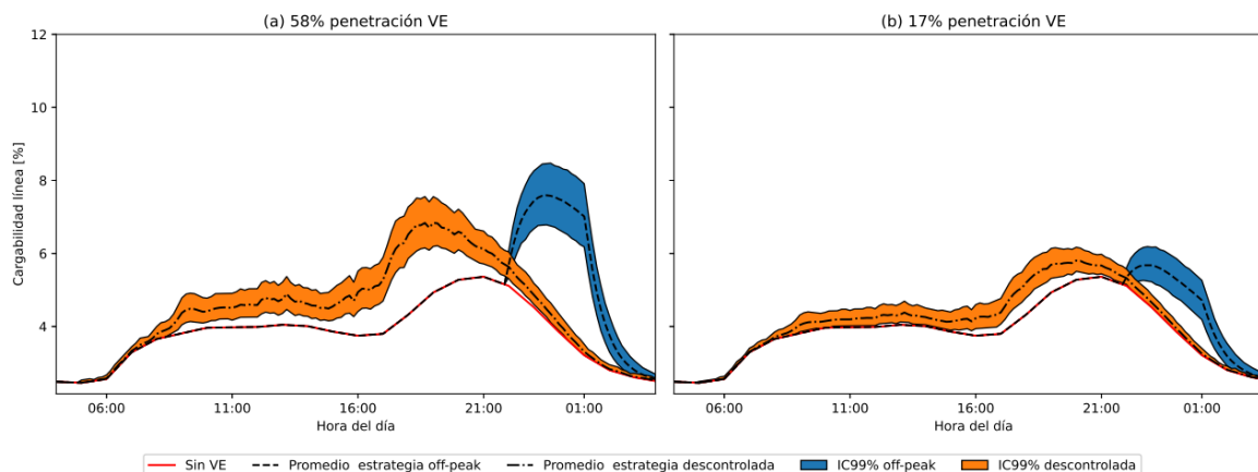
Figura 52: Comparación de la sobrecarga de la línea 4 cuando los VE tienen acceso a carga en todos los estados de estacionamiento. (Fuente: Elaboración propia).
