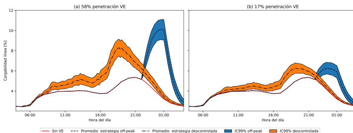
Figura 51: Comparación de la sobrecarga de la línea 4 cuando los VE tienen acceso solamente a cargadores domiciliarios y de CCR. (Fuente: Elaboración propia).
