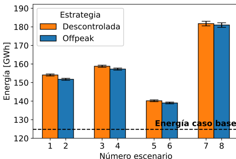
Figura 29: Comparación de la energía demandada diariamente producto de todos los eventos de carga para una penetración de VE del 58% (Fuente: Elaboración propia).
