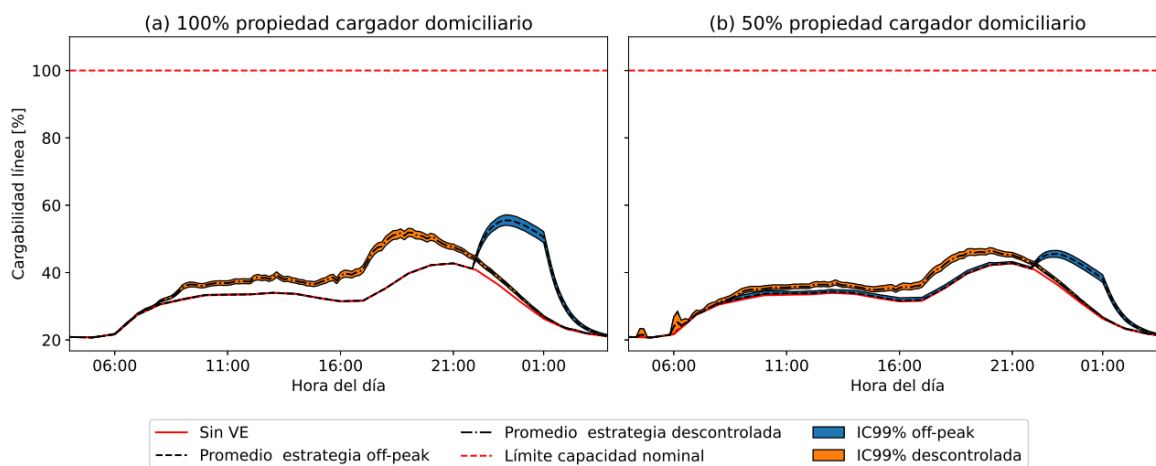
Figura 57: Comparación de la sobrecarga de la línea 2 cuando los VE tienen acceso a carga en todos los estados de estacionamiento. (Fuente: Elaboración propia).
