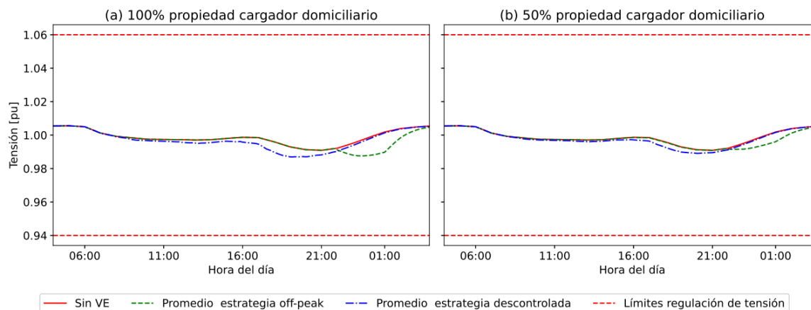
Figura 54: Comparación de la tensión eléctrica en el nodo 2 para un 58% de penetración cuando los VE tienen acceso solamente a cargadores domiciliarios y de CCR. (Fuente: Elaboración propia).
