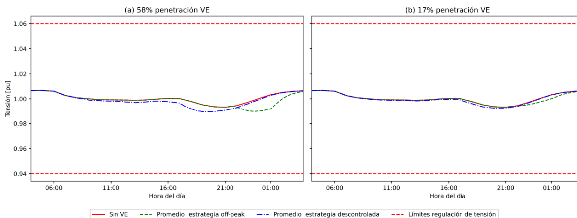
Figura 43: Comparación de la tensión eléctrica en el nodo 5 cuando los VE tienen acceso solamente a cargadores domiciliarios y de CCR. (Fuente: Elaboración propia).
