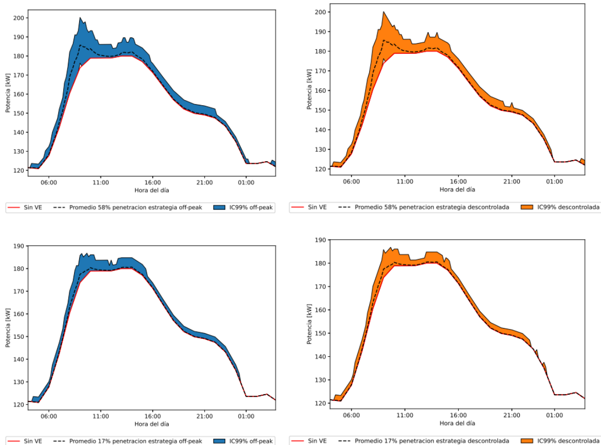
Figura 26: Comparación de la demanda eléctrica del lugar de trabajo ante distintos escenarios con 100% de propiedad de cargador domiciliario. (Fuente: Elaboración propia)
