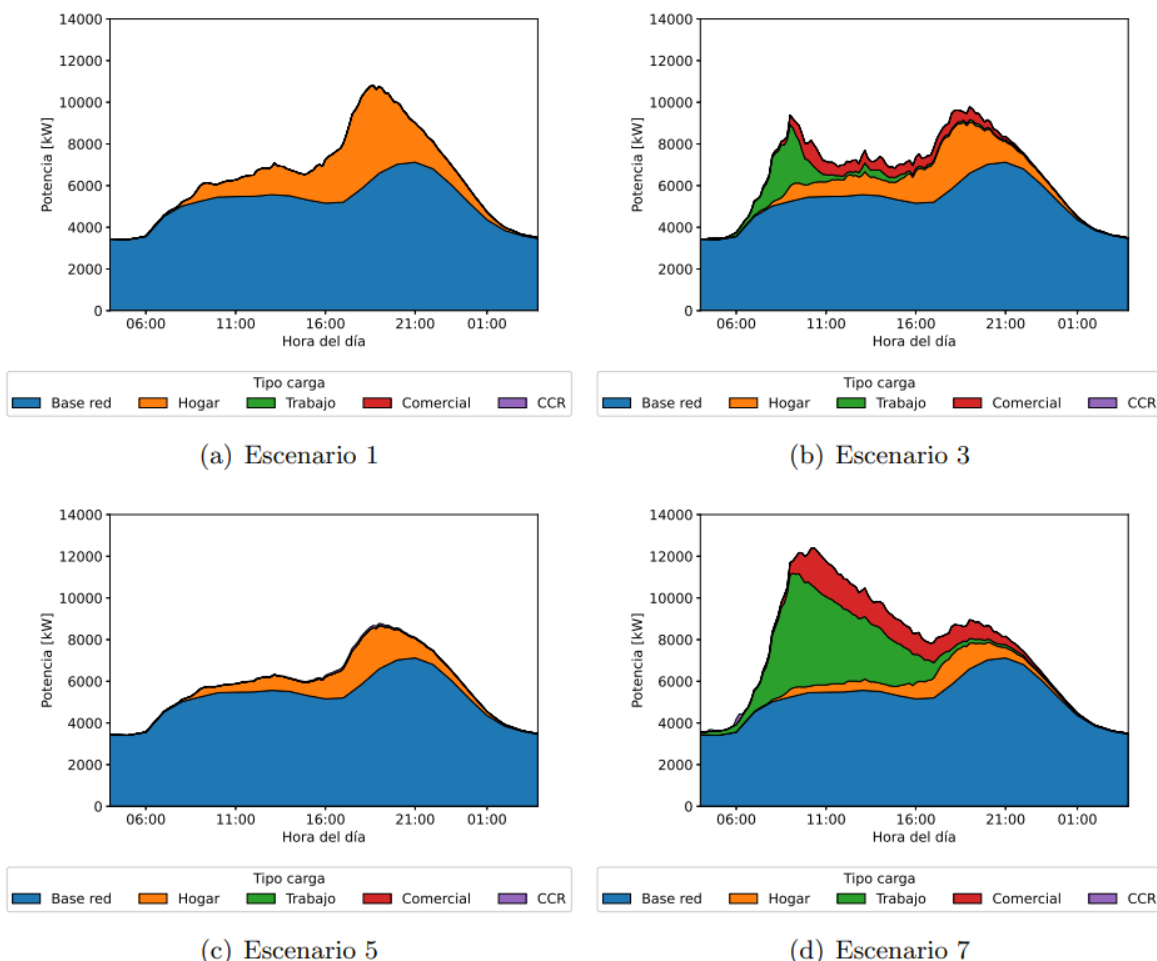
Figura 30: Comparación de escenarios 1, 3, 5 y 7 de la demanda eléctrica promedio de todos los eventos de carga bajo una estrategia descontrolada. (Fuente: Elaboración propia).
