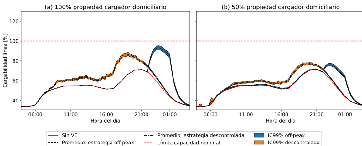
Figura 25: Comparación de la sobrecarga de la línea 1 cuando los VE tienen acceso a carga en todos los estados de estacionamiento. (Fuente: Elaboración propia).
