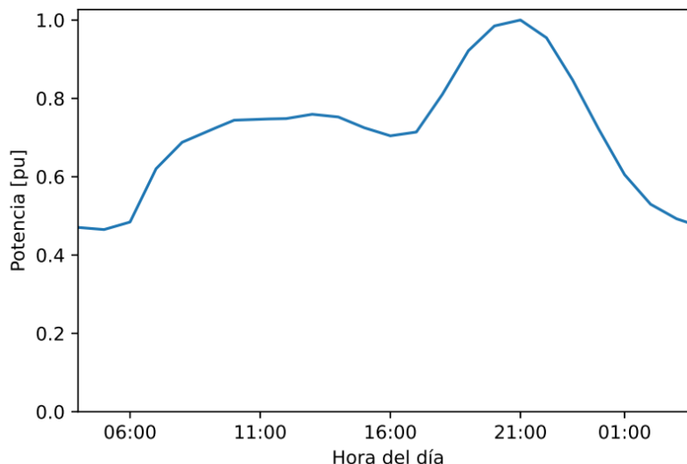
Figura 11: Perfil diario de demanda aplicado a todas las cargas de carácter domiciliario en el alimentador (Fuente: Elaborado con datos de SEC).
