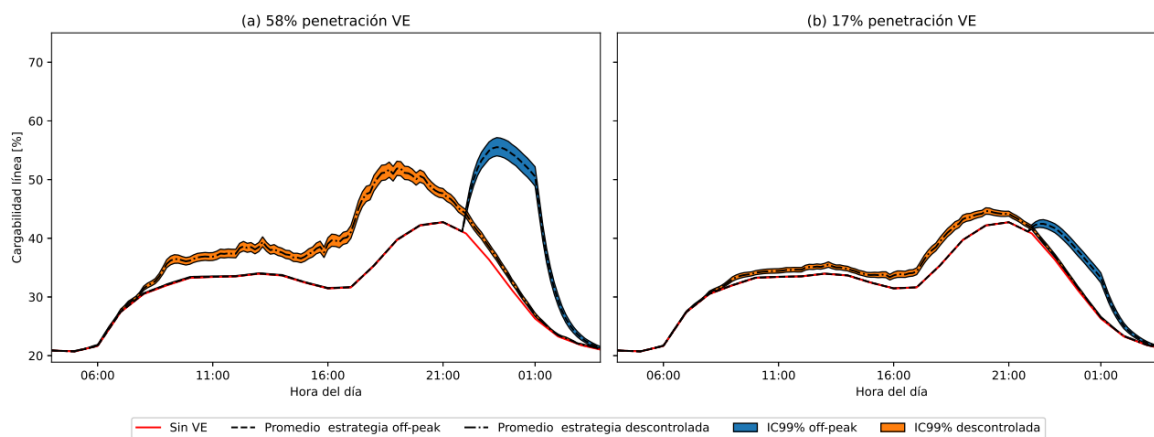
Figura 48: Comparación de la sobrecarga de la línea 1 cuando los VE tienen acceso a carga en todos los estados de estacionamiento. (Fuente: Elaboración propia).
