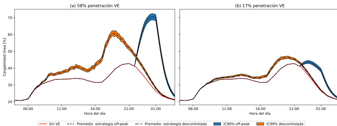
Figura 47: Comparación de la sobrecarga de la línea 2 cuando los VE tienen acceso solamente a cargadores domiciliarios y de CCR. (Fuente: Elaboración propia).
