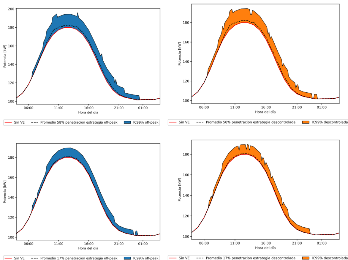
Figura 27: Comparación de la demanda eléctrica del lugar comercial ante distintos escenarios con 100% de propiedad de cargador domiciliario. (Fuente: Elaboración propia).
