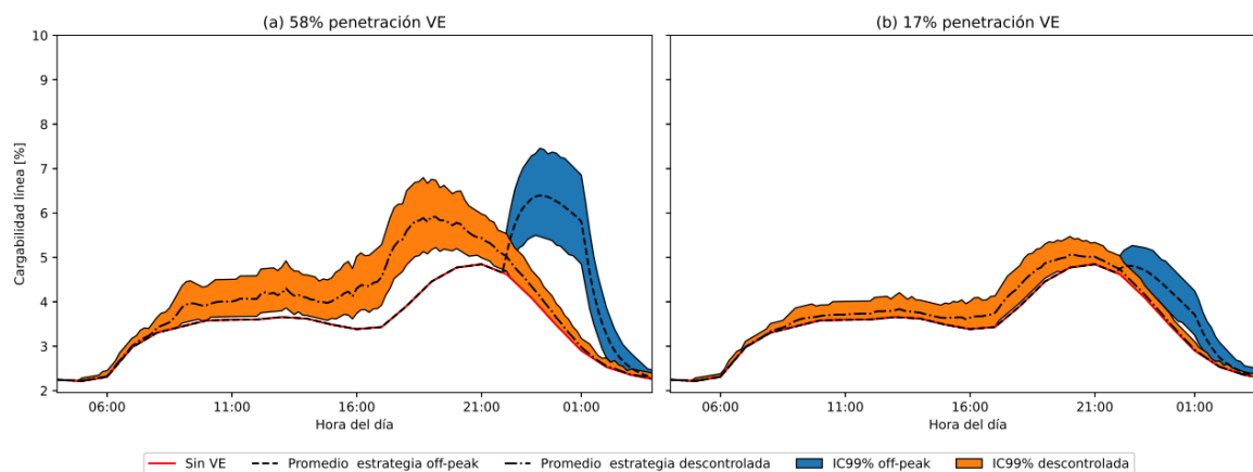
Figura 50: Comparación de la sobrecarga de la línea 3 cuando los VE tienen acceso a carga en todos los estados de estacionamiento. (Fuente: Elaboración propia).
