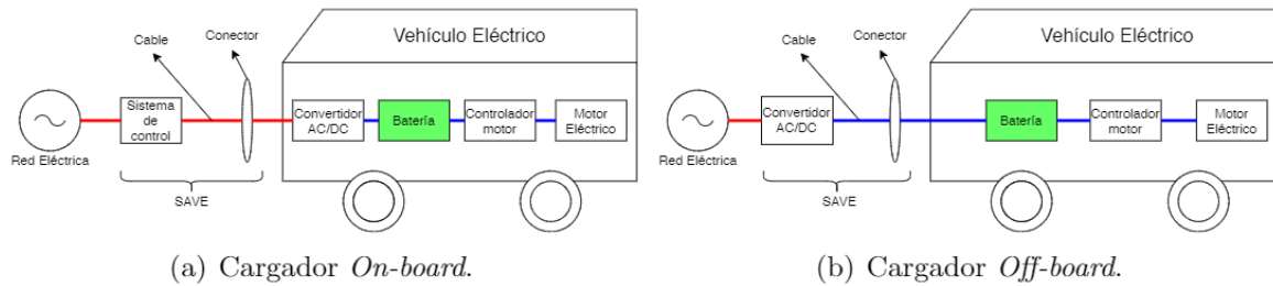
Figura 4: disposiciones típicas de un SAVE (Fuente: Adaptado de [20]).
