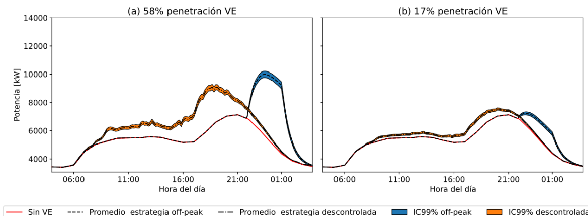
Figura 15: Comparación de la demanda eléctrica al principio del alimentador cuando los VE tienen acceso a carga en todos los estados de estacionamiento. (Fuente: Elaboración propia).
