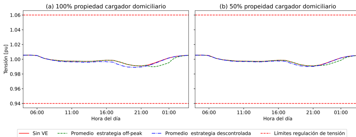
Figura 55: Comparación de la tensión eléctrica en el nodo 2 para un 58% de penetración cuando los VE tienen acceso a carga en todos los estados de estacionamiento. (Fuente: Elaboración propia).
