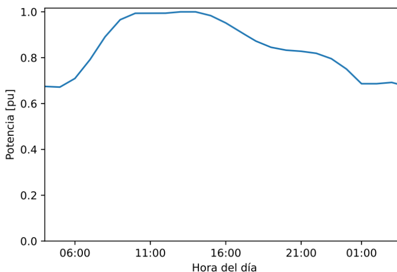
Figura 12: Perfil diario de demanda aplicado a todas las cargas de carácter comercial en el alimentador. (Fuente EPRI [60])
