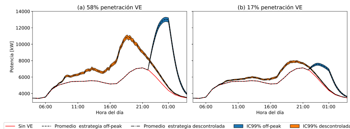
Figura 14: Comparación de la demanda eléctrica al principio del alimentador cuando los VE tienen acceso solamente a cargadores domiciliarios y de CCR. (Fuente: Elaboración propia).
