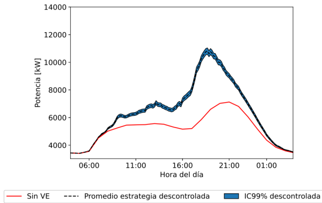
Figura 58: Demanda eléctrica producto de todos los eventos de carga de la flota de VE simulada para el escenario 1. (Fuente: Elaboración propia).
