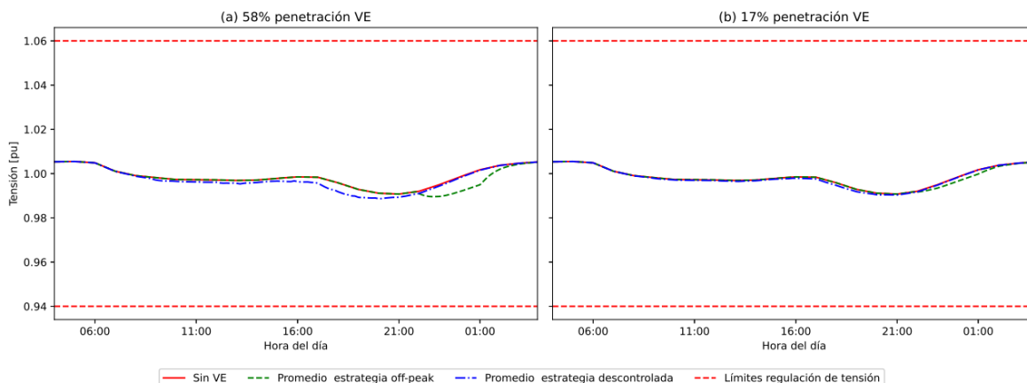
Figura 42: Comparación de la tensión eléctrica en el nodo 4 cuando los VE tienen acceso a carga en todos los estados de estacionamiento. (Fuente: Elaboración propia).
