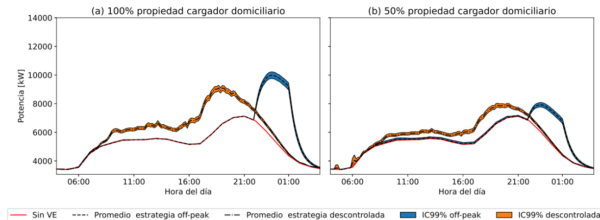
Figura 21: Comparación de la demanda eléctrica en cabecera del alimentador con un 58% de penetración, considerando que los VE tienen acceso a carga en todos los estados de estacionamiento. (Fuente: Elaboración propia).
